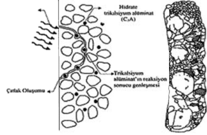
Şekil 1. Sülfatın betona teması
